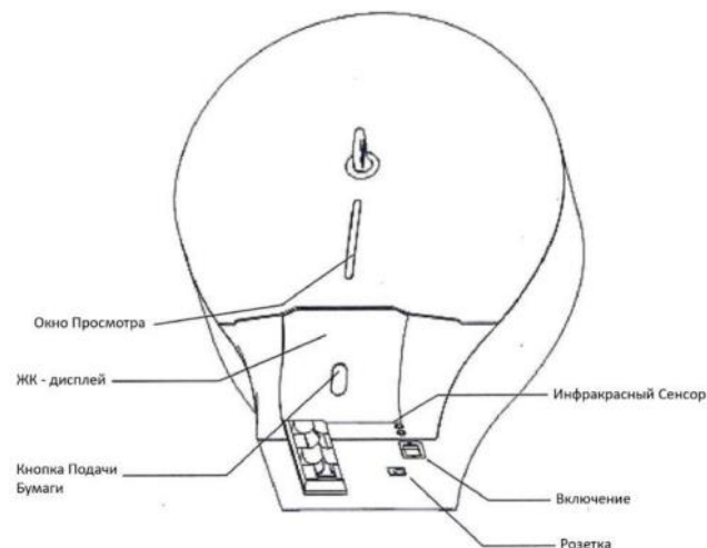
Рис.2. Внешняя конструкция
