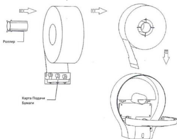
Рис.3. Установка бумаги
