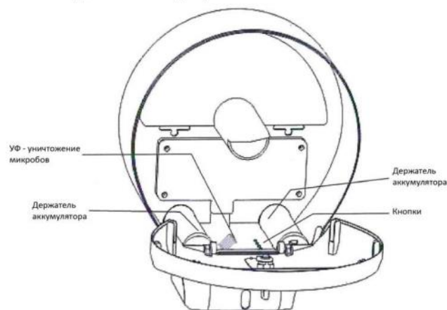
Рис.2. Внешняя конструкция
